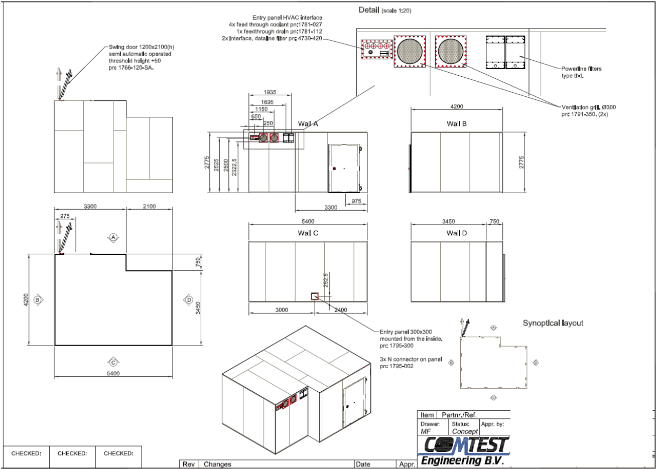
Plan de réalisation d’une cage de faraday en acier avec filtration
